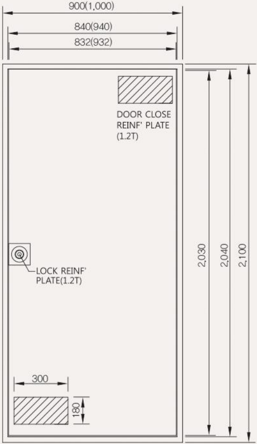
방화문 정면도
