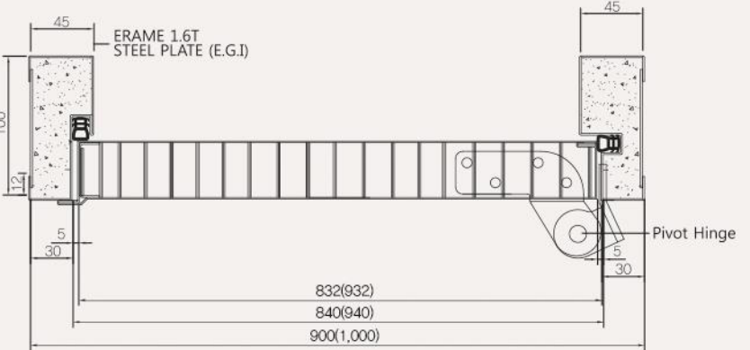
수평단면도
