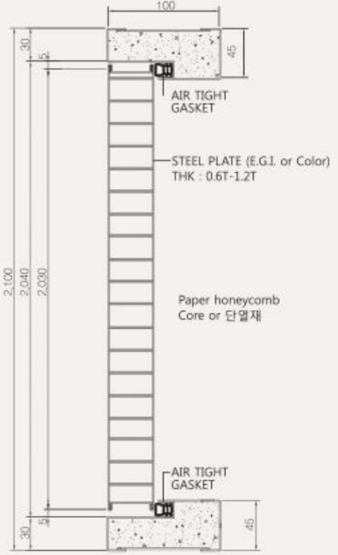
수직단면도
