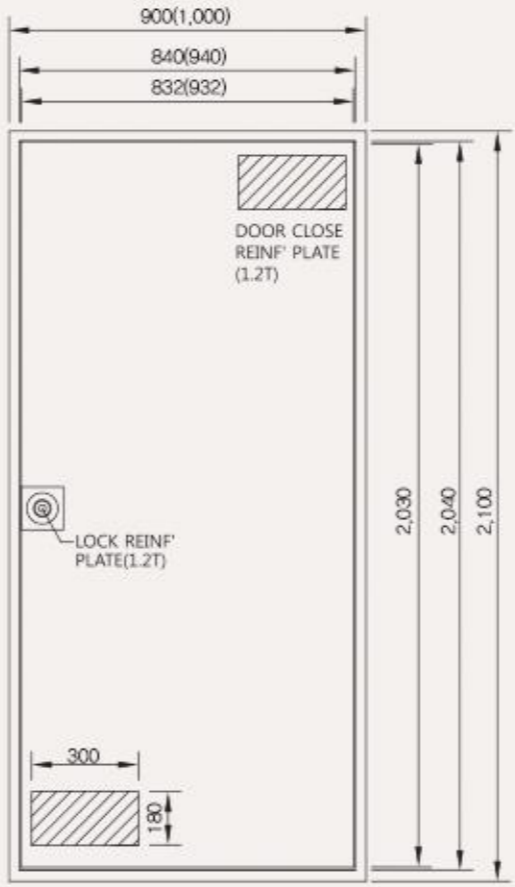
방화문 정면도
